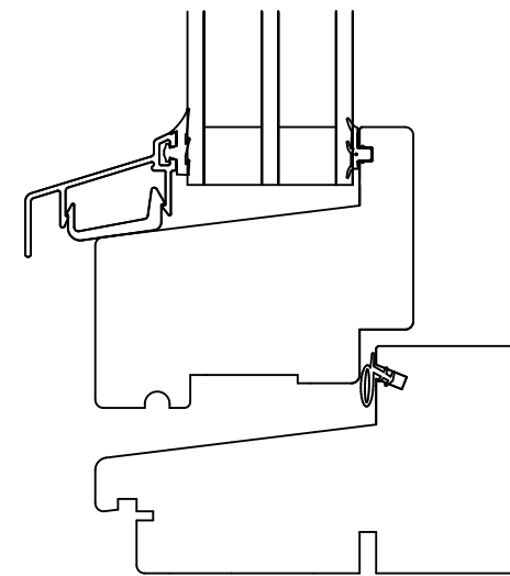
SEKTION A SKALA 1:2
