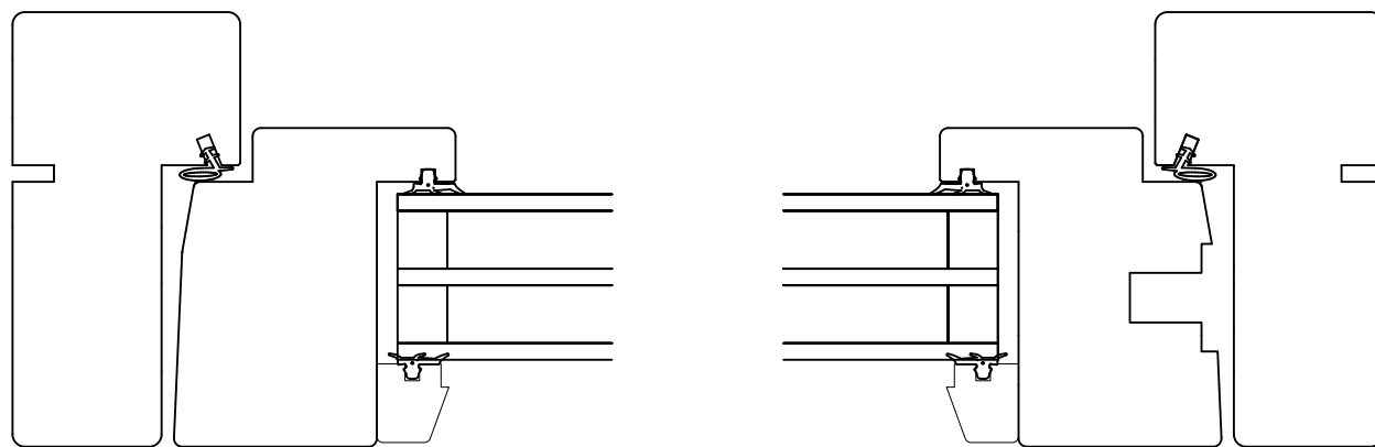
SEKTION B SKALA 1:2
