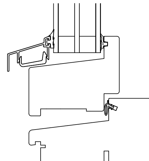
SEKTION A SKALA 1:2
