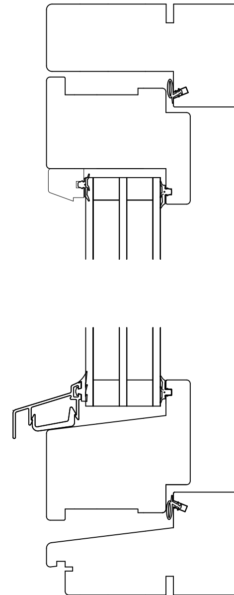
SEKTION A SKALA 1:1
